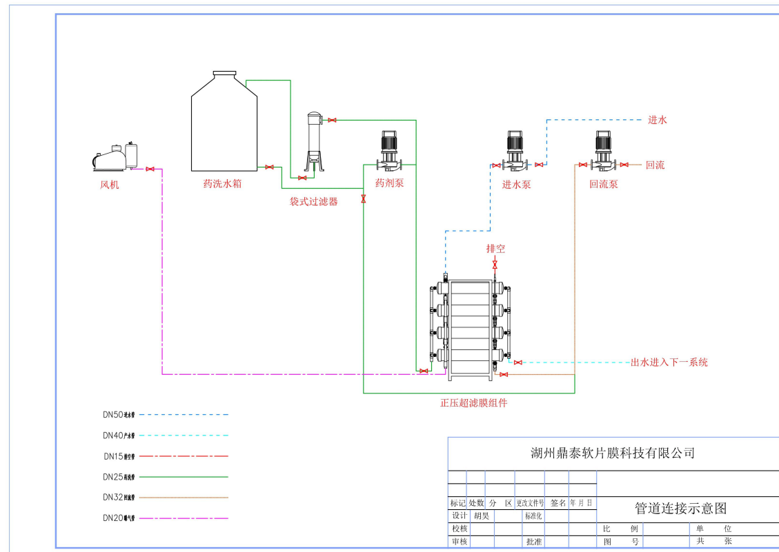
正压超滤膜系统示意图
