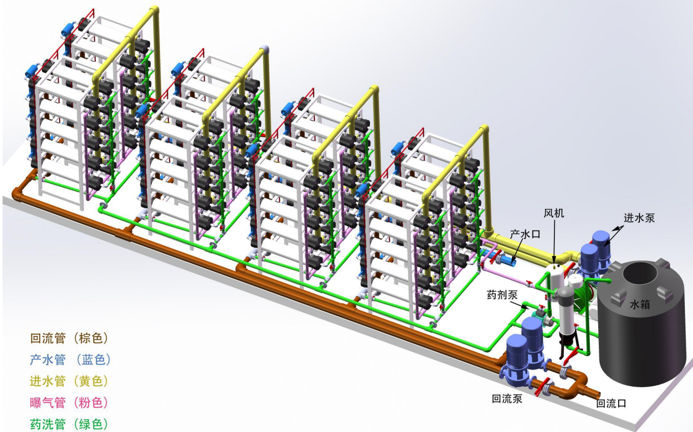
正压超滤膜系统布置图
