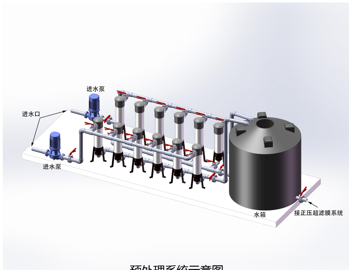
预处理系统示意图
