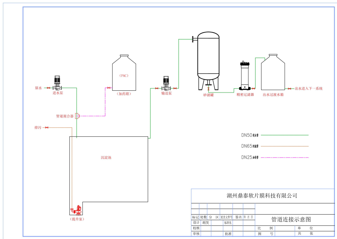
预处理系统示意图
