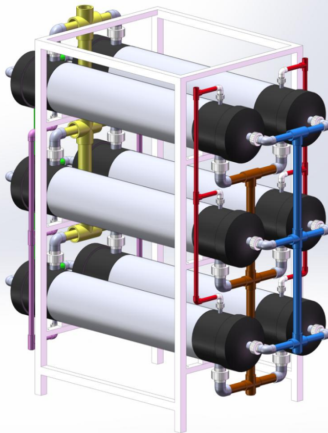
YL-6E2膜组件示意图
