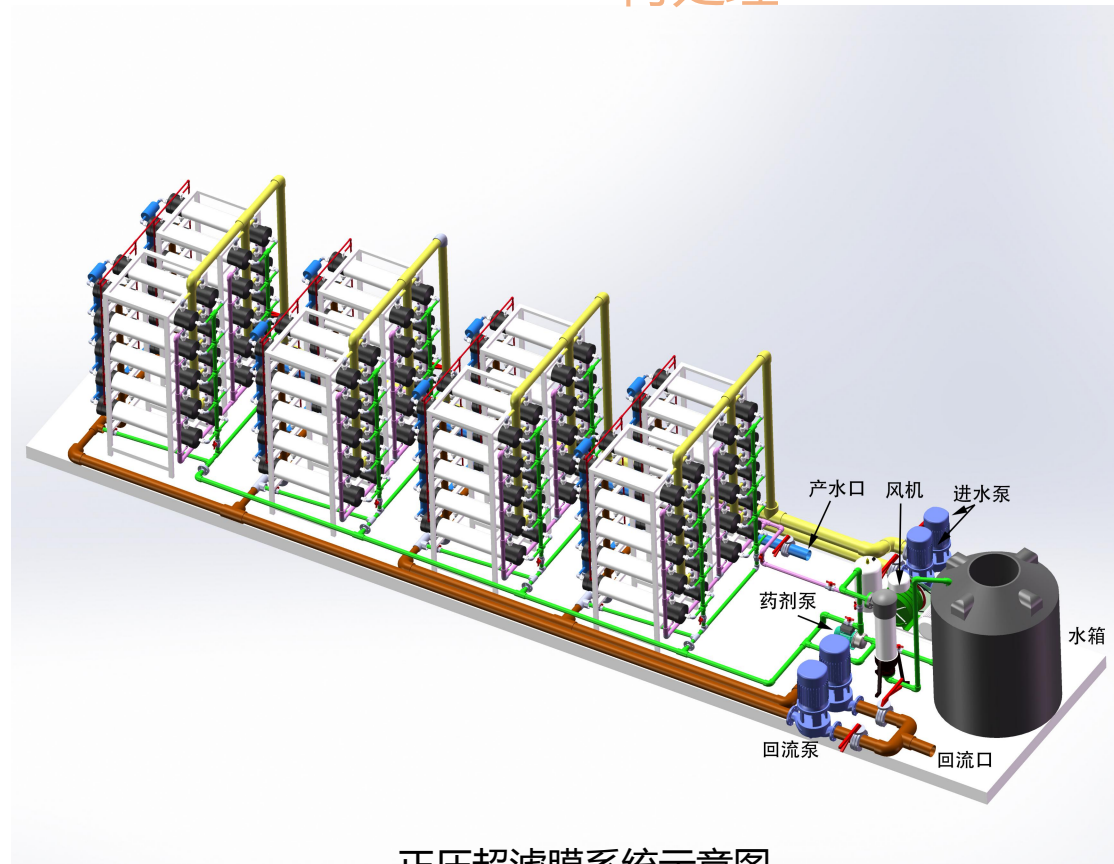
正压超滤膜系统示意图
