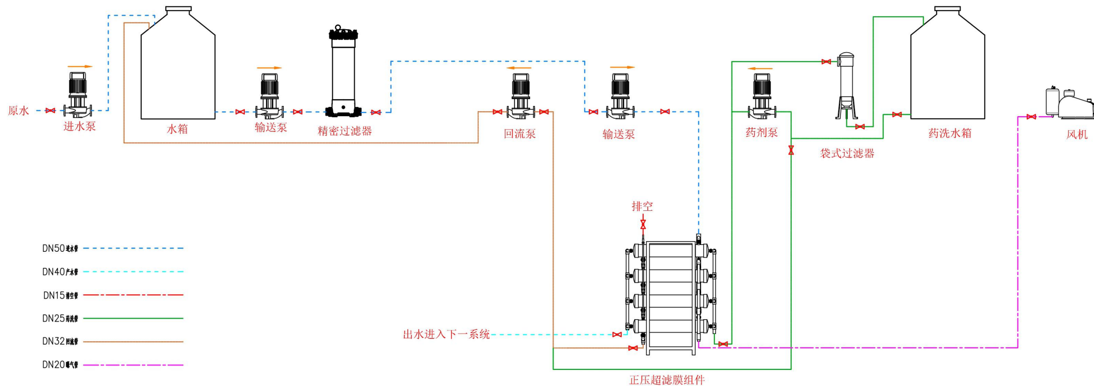
预处理系统示意图
